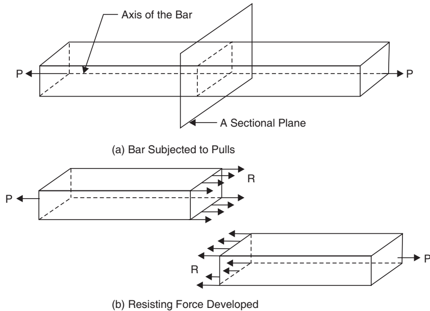
Fig. 5. Tensile Stresses
